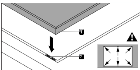
Abb. 9.30 Höhenausgleichsplatten einlegen
