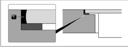
Abb. 9.45 Silikondichtmasse bei flächenbündiger Montage
