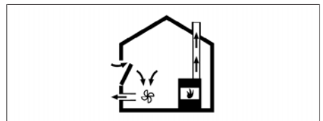
Abb. 9.2 Abluftmontage – korrekt
