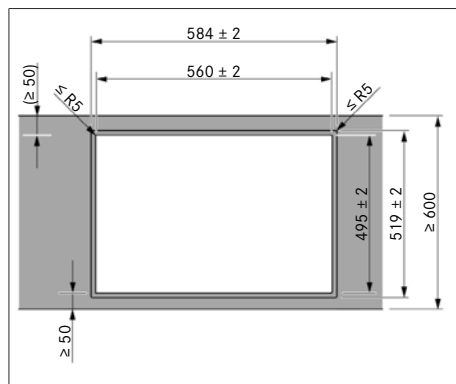
Abb. 9.9 Ausschnittsmaße für flächenbündige Montage
