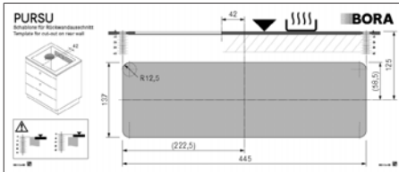
Abb. 9.24 Schablone für Rückwandausschnitt
