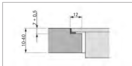
Abb. 9.10 Falzmaß für flächenbündige Montage
