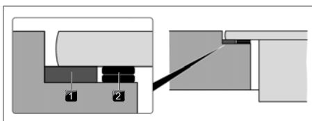
Abb. 9.31 Höhenausgleichsplatten
