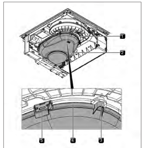
Abb. 7.3 Luftführungsgehäuse
