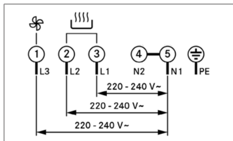
Abb. 9.35 Anschlussschema Dreiphasen-Anschluss
