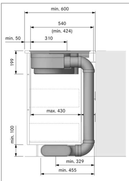
Abb. 9.11 Einbaumaße bei Abluft, Arbeitsplattentiefe 600 mm
