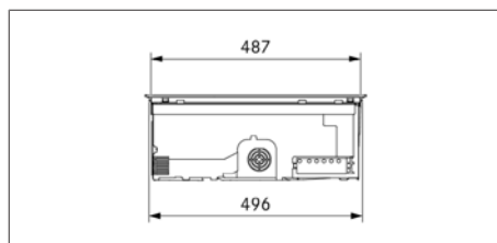
Abb. 3.6 Seitenansicht PURSU
